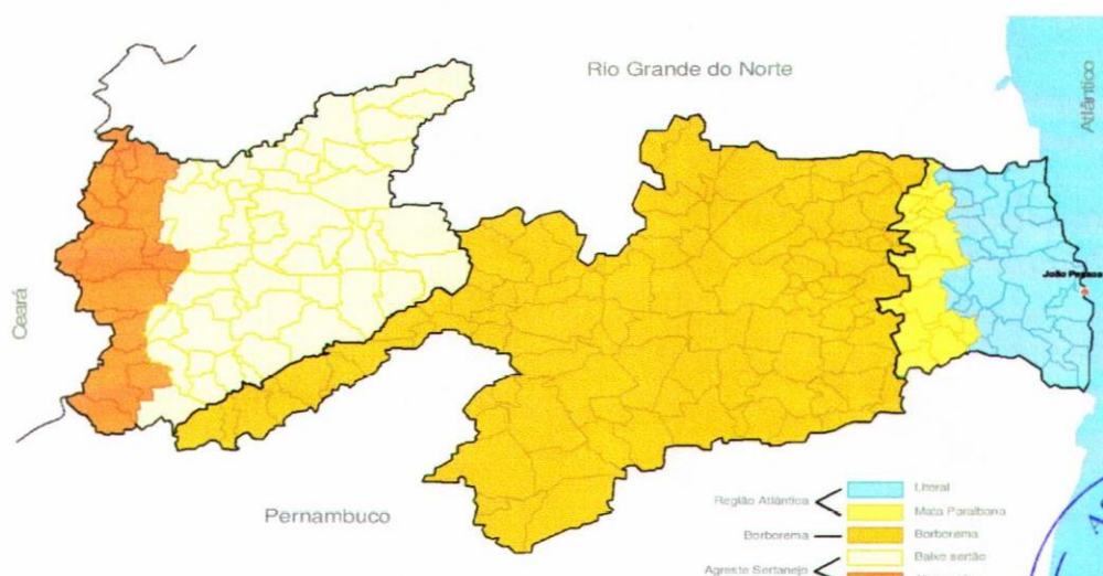
Mapa 1 - Geologia do Estado da Paraíba
